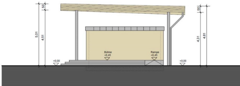
Ansicht von rechts M11100
