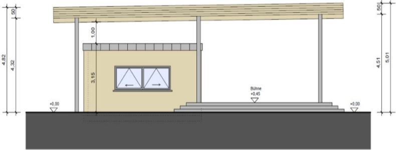
Ansicht Vorderseite M11100
